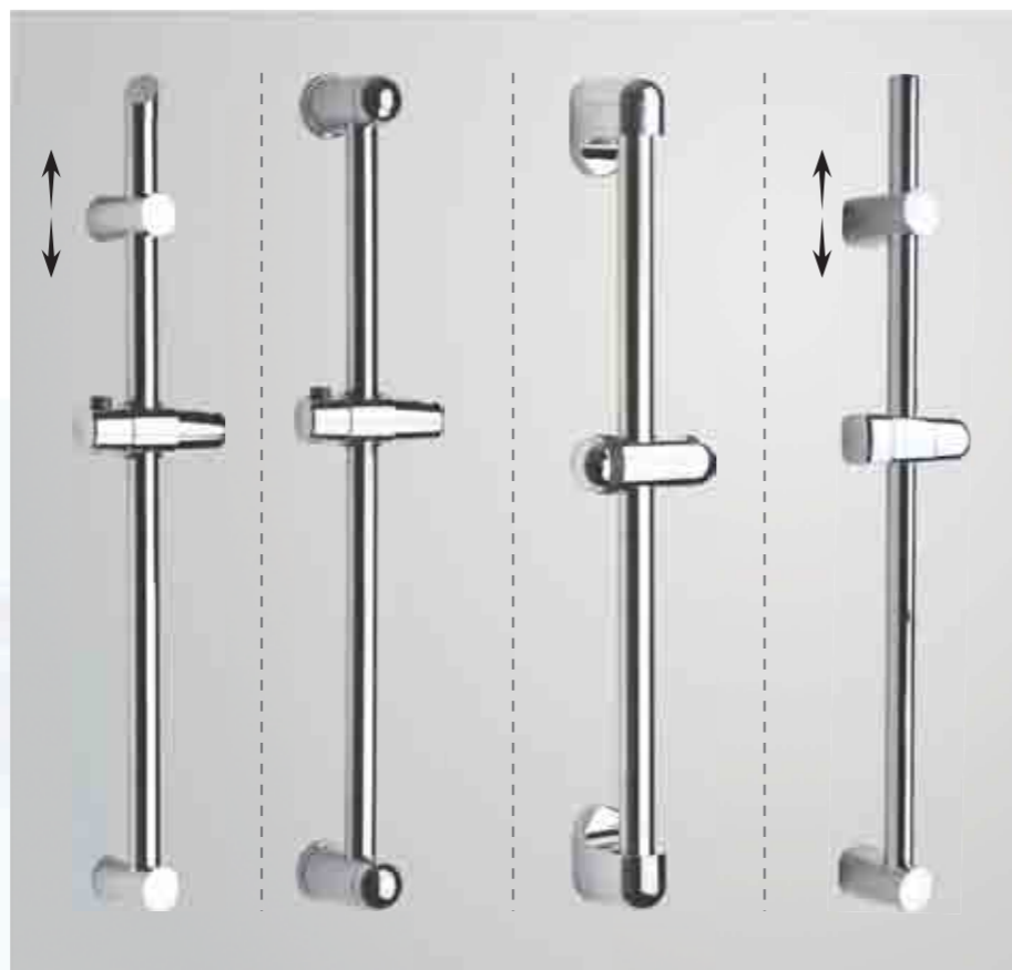
B723 Φ25*700mm B724 Φ25*600mm B725 Φ30*600mm B726 Φ25*700mm
